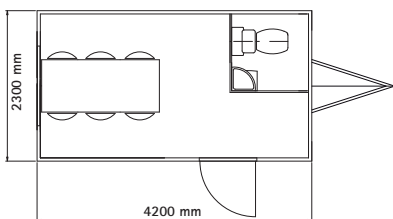
Model 420 - 6 personers spisevogn
