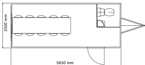
Model 565 - 10 personers spisevogn
